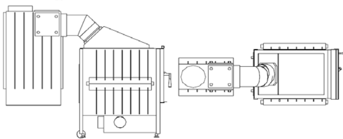
Odladěná verze výměníku Kobok - VERTIKAL KPL 75 - 4kW , VERTIKAL KPL 100 5kW - výstupní teplota spalin 160°C
